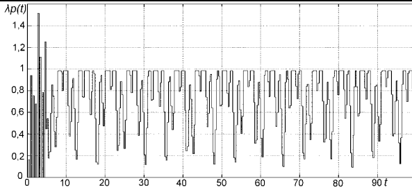
Рис. 7 – Перехідна характеристика систем управління потоками трафіку на основі оптимального по швидкодії регулятора.
