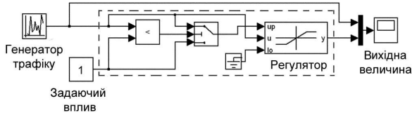
Рис. 1 – Модель систем управління потоками трафіку на основі апаратного регулятора.
